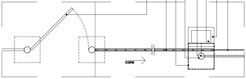
DETALHE 05 ESCALA 1/20 CIS/CS/CSM em ferrozinco
