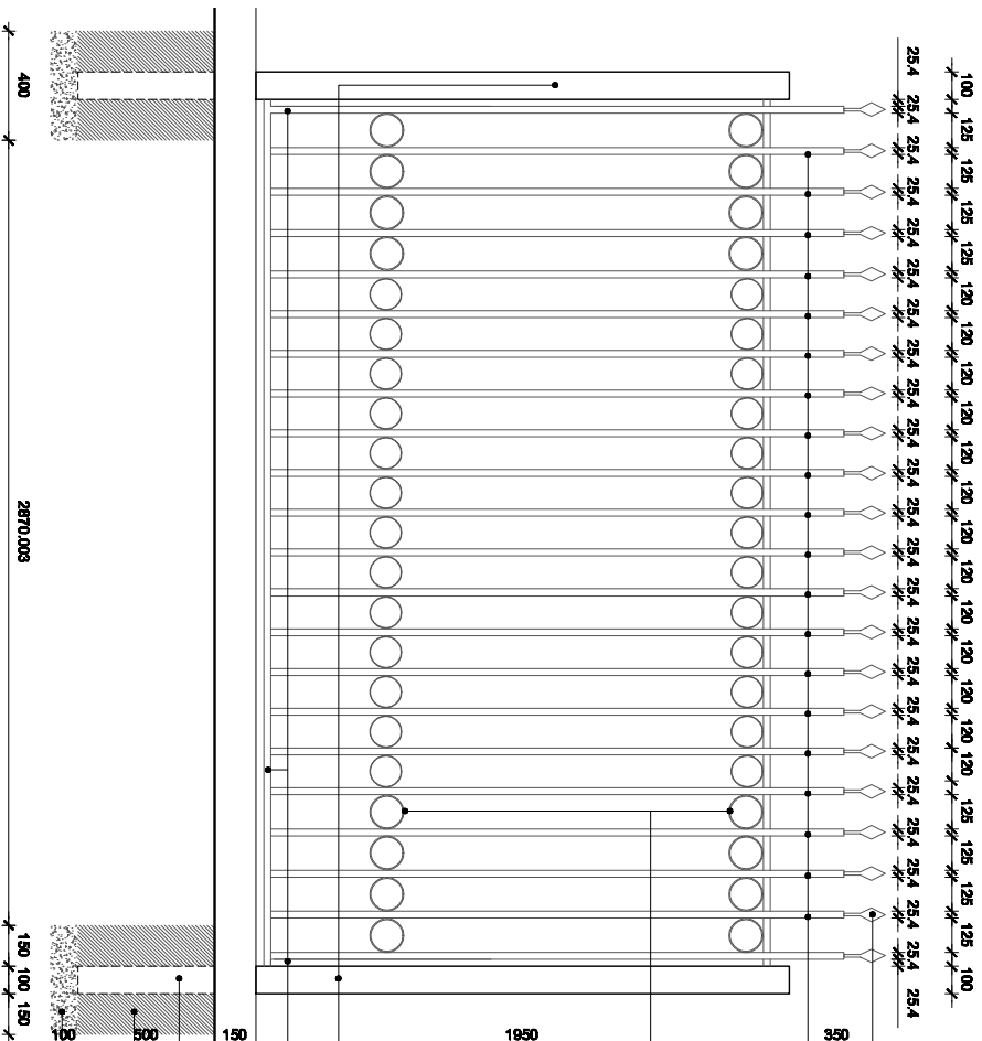
DETALHE 04 ESCALA 1/20 CIS/CS/CSM em ferrozinco
