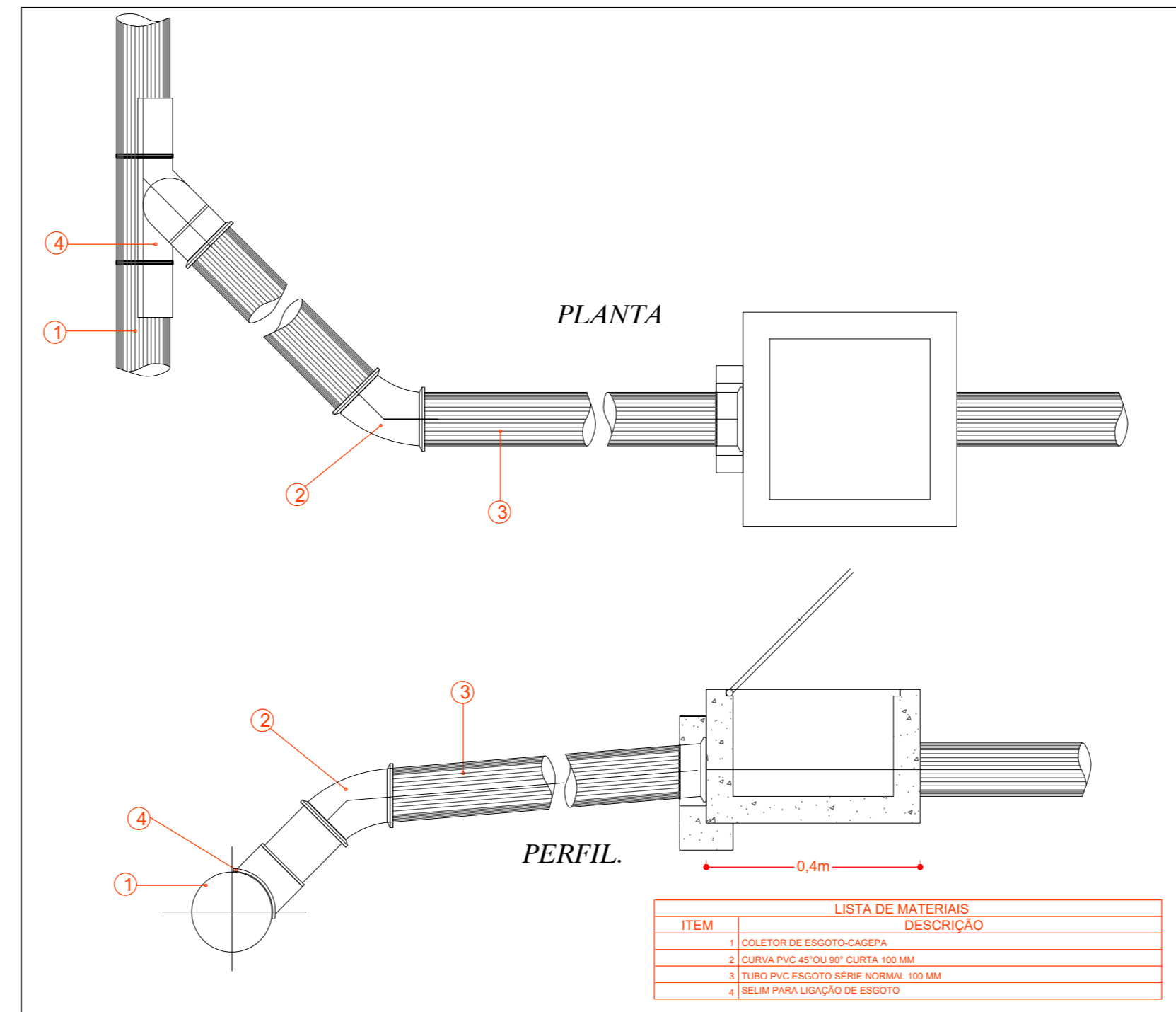
D2 - LIGAÇÃO COM COLETOR DE ESGOTO SEM ESCALA
