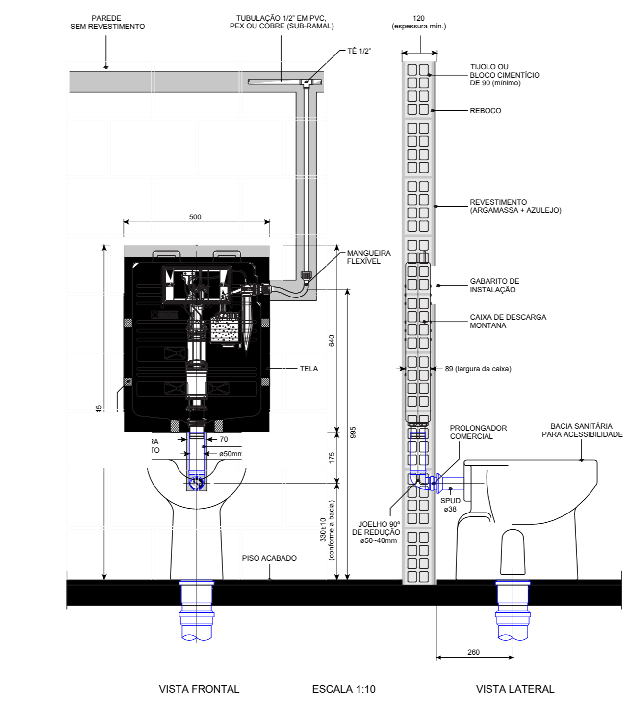
CAIXA MONTANA ESCALA 1/10
