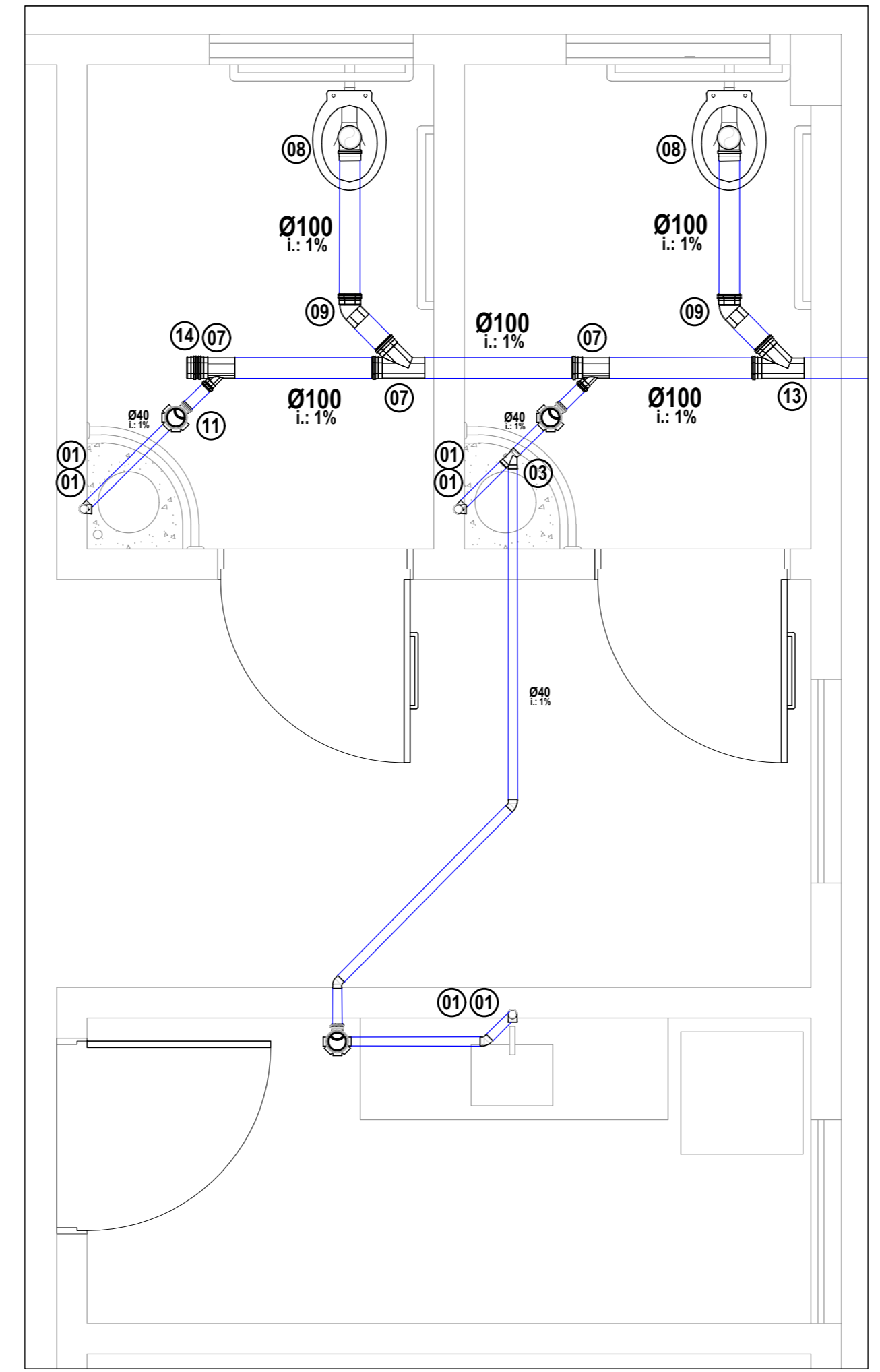
PLANTA BAIXA - ESGOTO BANHEIROS ESCALA 1/25
