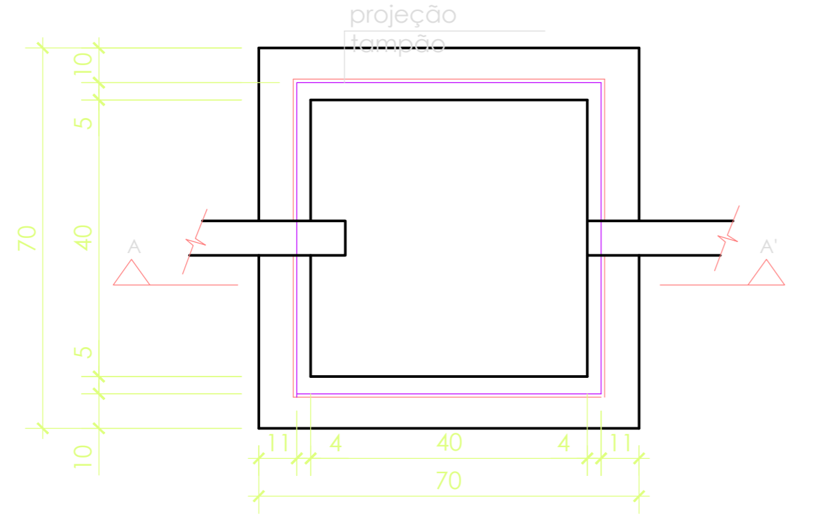
D1-CAIXA DE INSPEÇÃO SEM ESCALA
