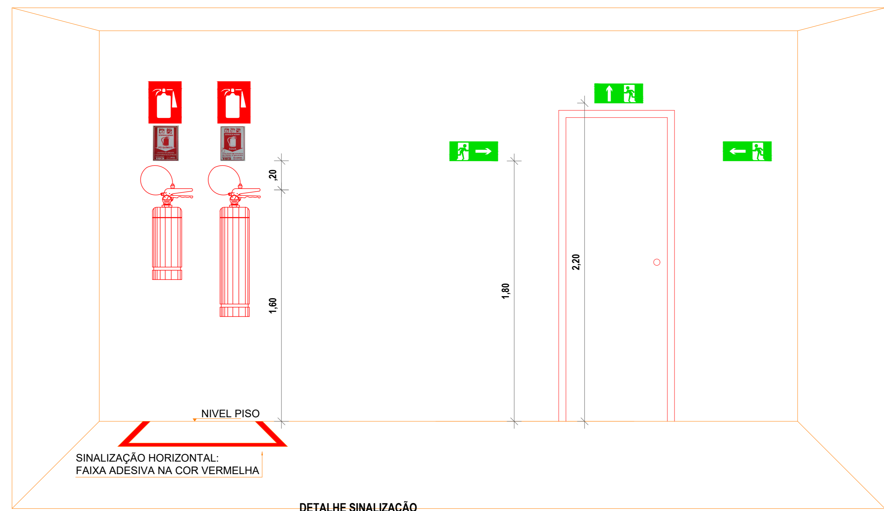
DETALHE SINALIZAÇÃO SEM ESCALA
