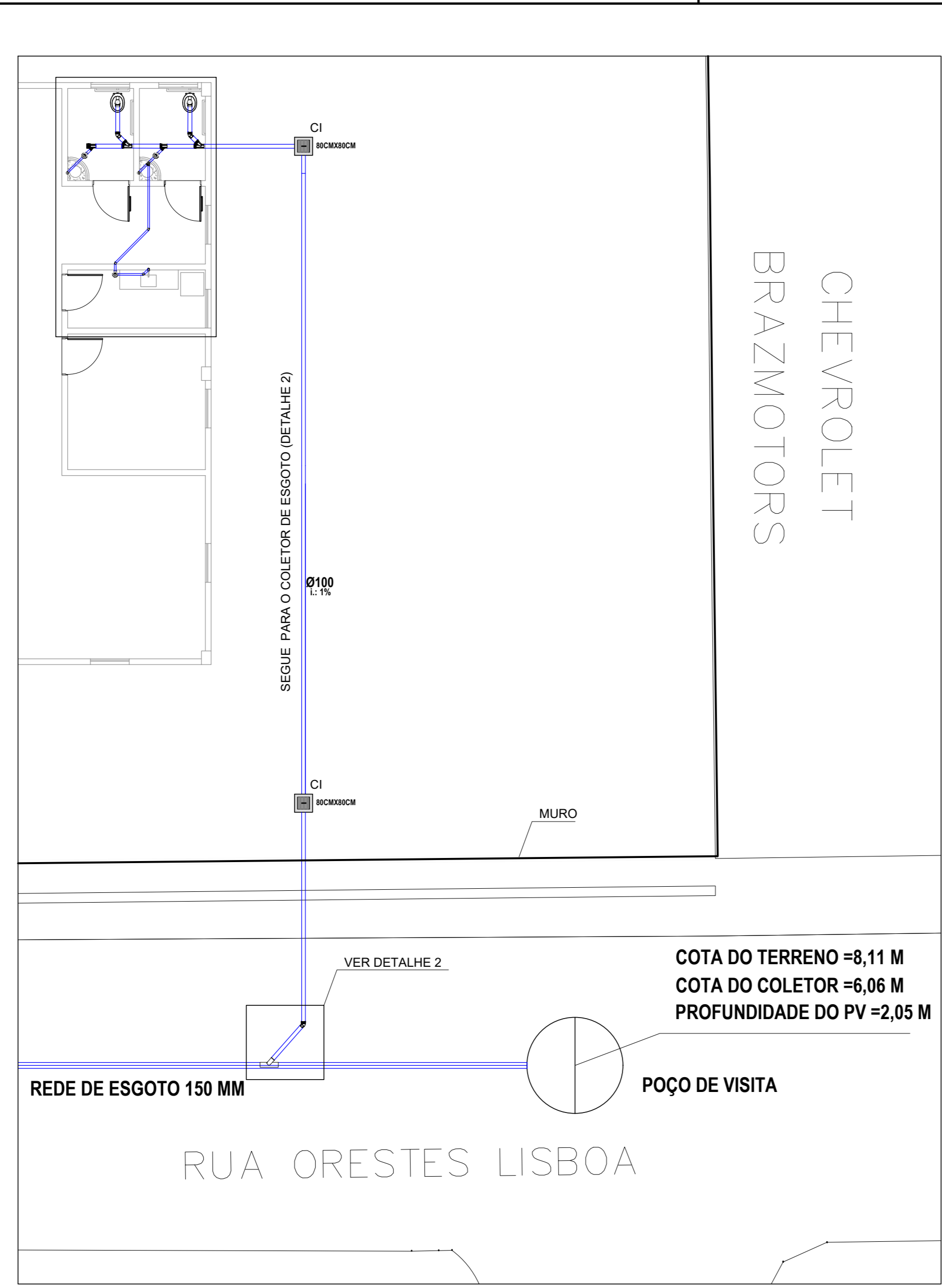
PLANTA BAIXA - ESGOTO ESCALA 1/100
